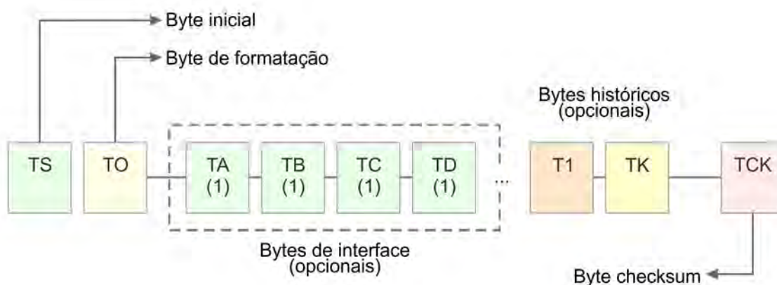
Figura 3.4b - Conteúdo do ATR.
