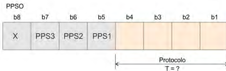
Figura 3.5b - Conteúdo do byte PPS0.
