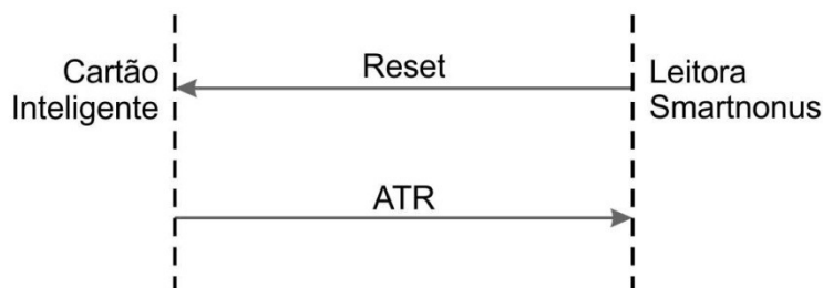
Figura 3.4a - Após o Reset, o cartão envia uma resposta ATR.
