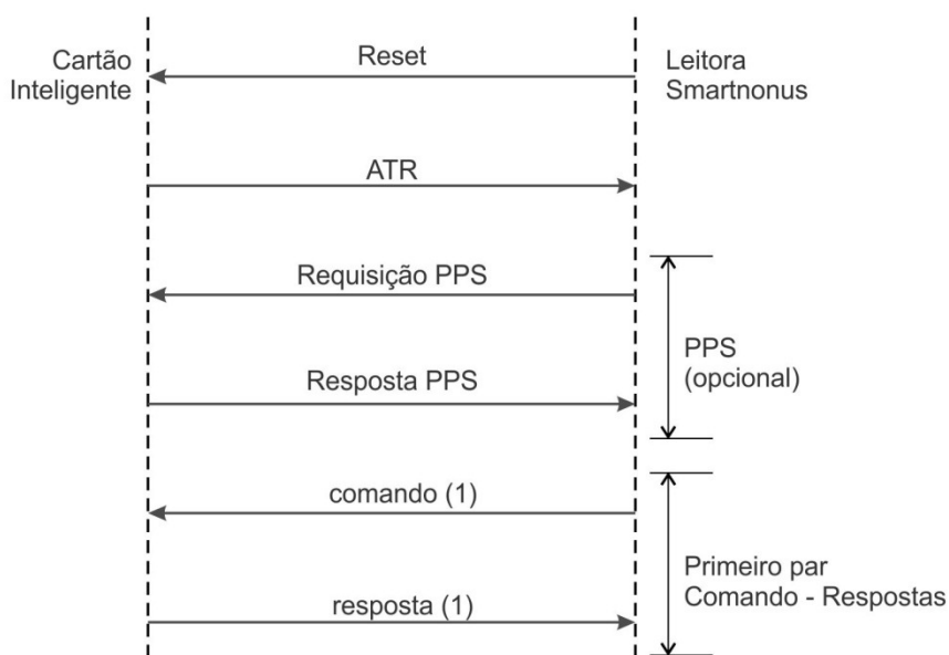
Figura 3.5a - Caso preciso, o comando PPS é executado logo após o ATR, antes do primeiro par comando-resposta.
