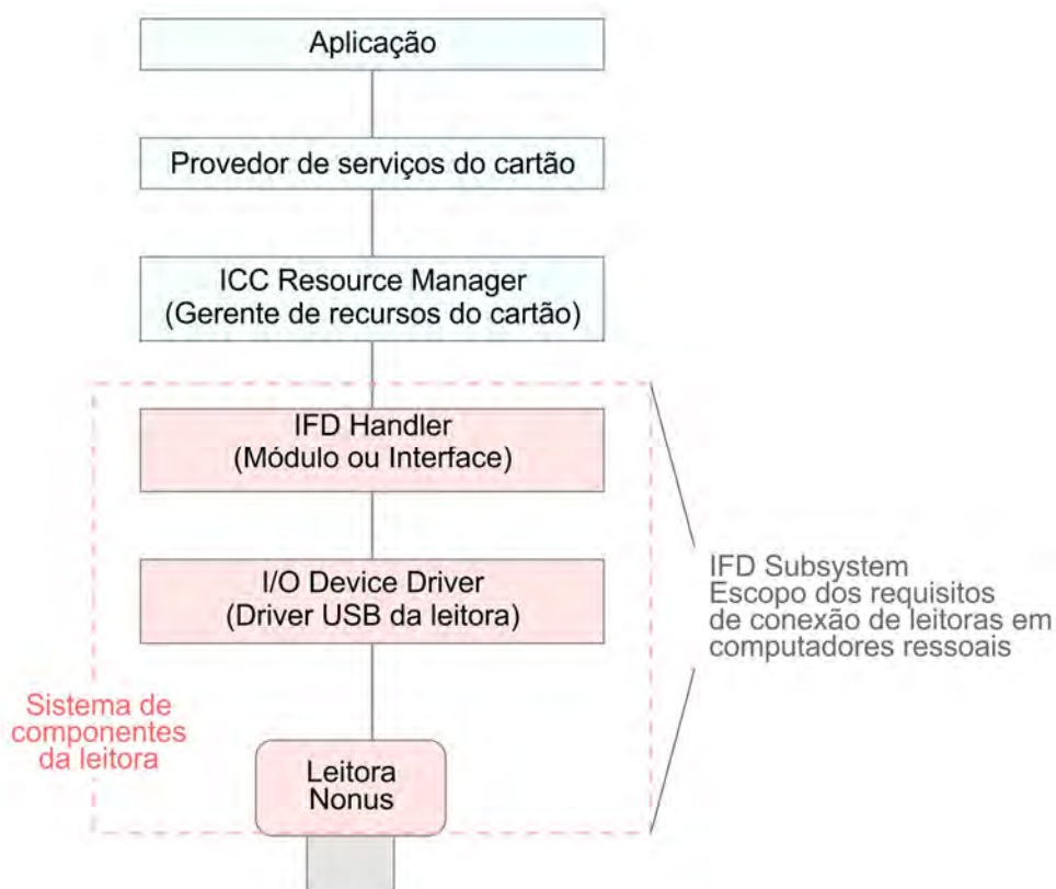
Figura 4a – Arquitetura PC/SC
