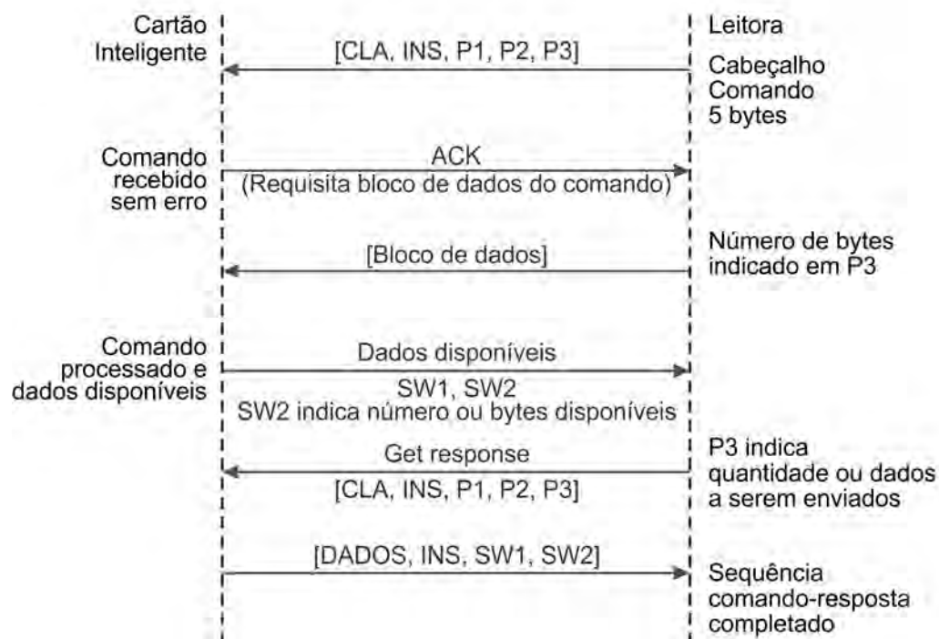
Figura 3.6.1 - Caso mais extenso de instrução no protocolo T=0.
