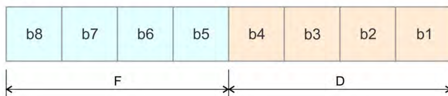
Figura 3.4c - Conteúdo do byte TA.
