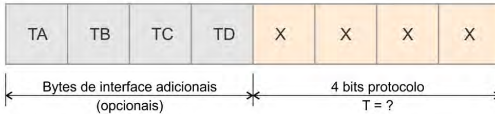
Figura 3.4d - Conteúdo do byte TD.
