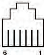
Conector RJ fêmea
