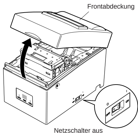
Abb. 5-8 Druckerabdeckung öffnen.
